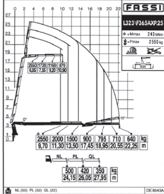
Lastdiagramm Kran mit Verlängerung
