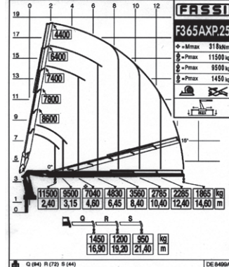
Lastdiagramm Kran ohne Seilwinde
