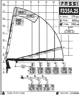
Lastdiagramm Kran mit Verlängerung
